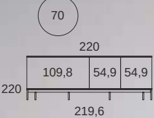
231 / CALIFORNIA-BLANCO MATE Yours - ancho: 220cm / alto: 180cm / fondo: 45cm
