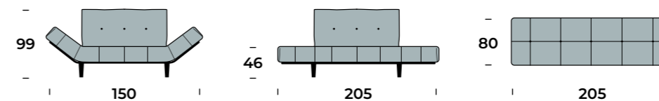
Sofá-cama cerrado 150x99x83 | Sofá-cama abierto 205x99x83 | Sistema bisagra multiposiciones en ambos lados | Bastidor de metálico con 7 lamas de madera | Asientos de espuma de poliuretano D28kg/m3 | Respaldo fibra hueca siliconada | Patas de madera de altura 24cm
